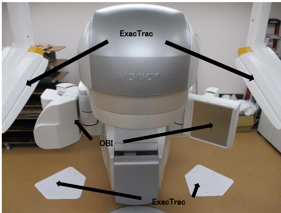
TrueBeam STxに実装される OBI(CBCT)と ExacTrac
